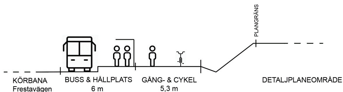
Schematisk sektion för Frestavägens östra sida vid framtida busshållplats, med eventuellt regionalt cykelstråk.
