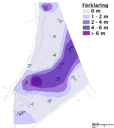
Lermäktighet från tolkningen av MUR (Tyréns 2019-12-05)
