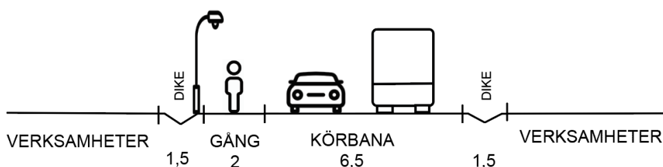
Schematisk sektion för ny intern gata.
