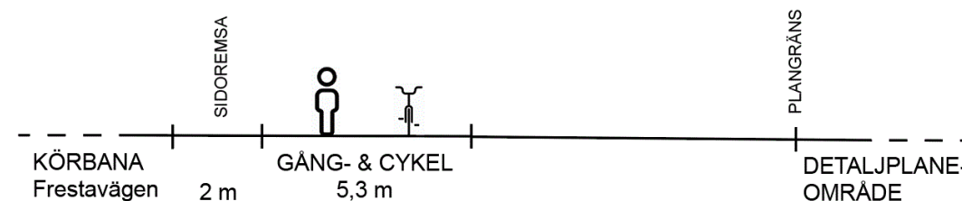
Schematisk sektion för Frestavägens östra sida i södra delen av planområdet, med eventuellt regionalt cykelstråk.
